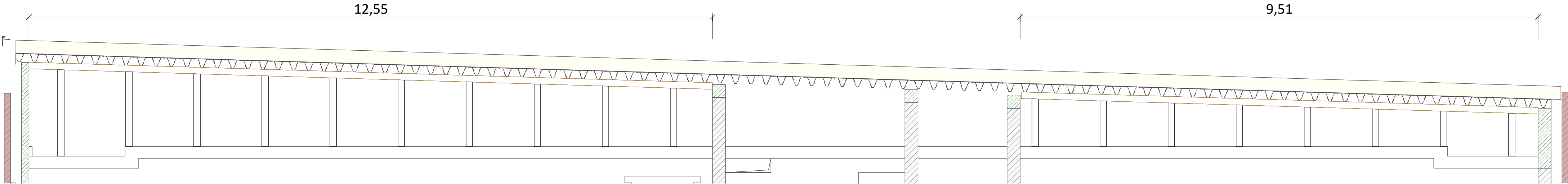
Randbalken auf Pfosten als Trapezblechauflager in Achse 2
