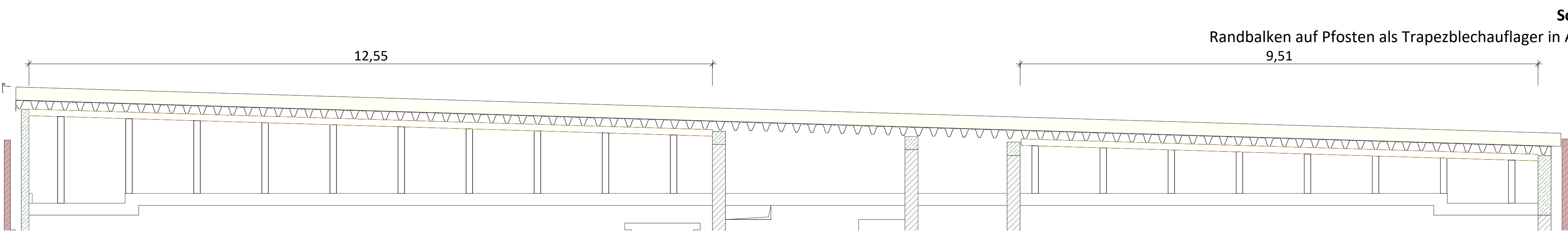
Fachwerkträger über Schulungsraum Pos.: 50s (20/14 + 18/14 + 10/14 cm)
